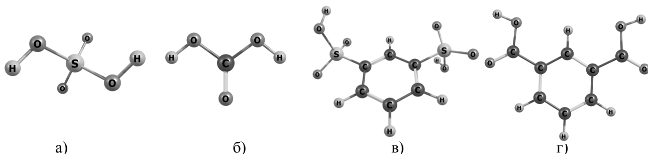
Рис. 1. Наиболее устойчивые конформеры кислот: а) серная; б) 1,3 –БДСК;в) угольная; г) 1,3-БДКК
