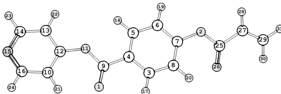
Рис.2. Нумерация атомов в молекуле
