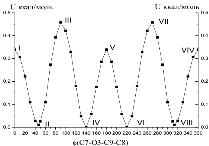
Рис. 1. Потенциальная функция внутреннего вращения пиридинового фрагмента вокруг связи С-О в молекуле 1-окси[4-карбокси(4'-пиридинил)]пропеноата
